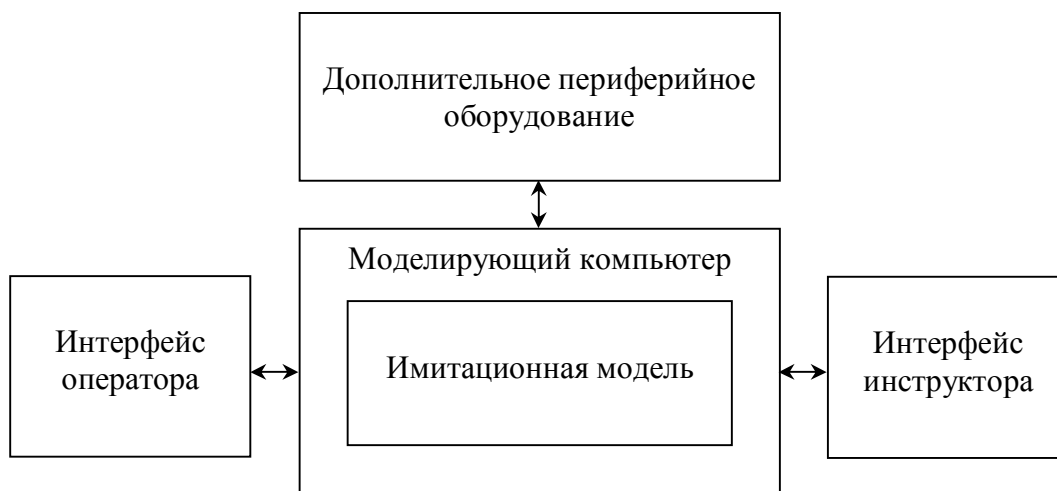
Рисунок 1 – Структура тренажера
